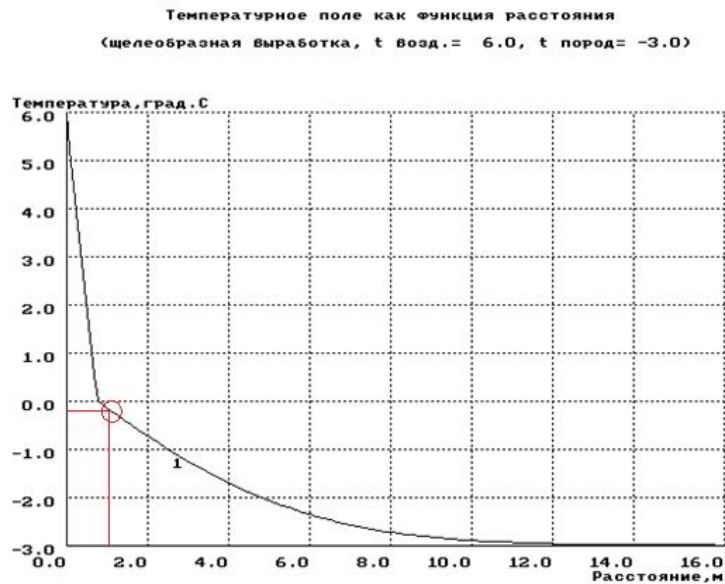
Рисунок 1. Температурное поле горных пород при использовании конвейеров
